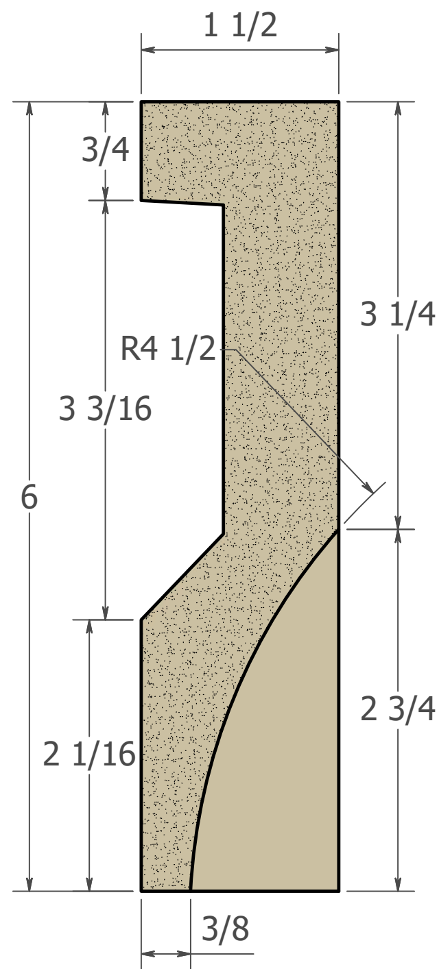
SECTION A-A SCALE 1 : 1
