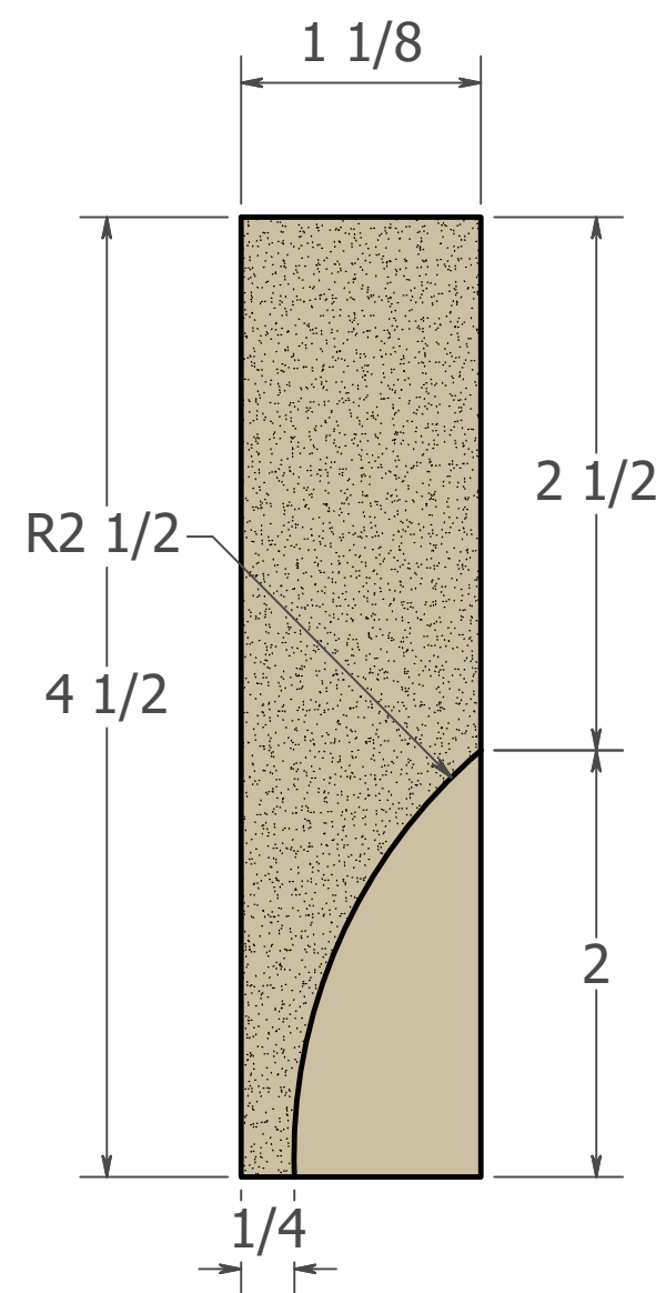
SECTION A-A SCALE 1 : 1
